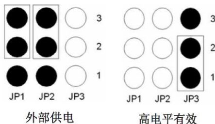
图 12. 跳线 JP1, JP2, JP3 的设置
